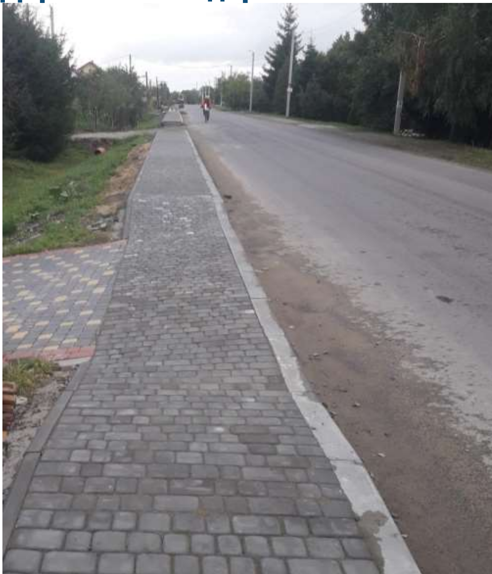
Влаштування тротуарів по вул.Артищівській, м. Городок
